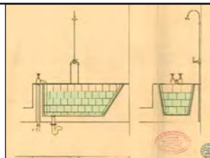
Plan van de badkuipen
